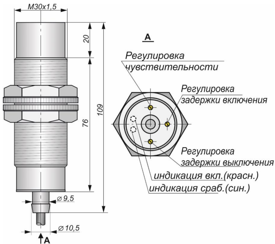
Габаритный чертеж
