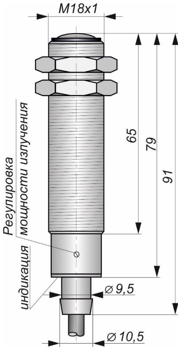
Габаритный чертеж
