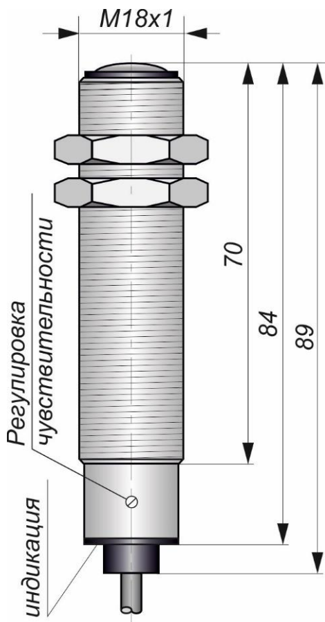
Габаритный чертеж
