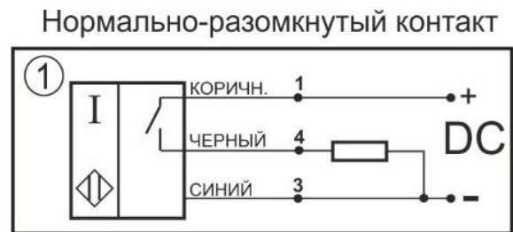
Схема соединения
