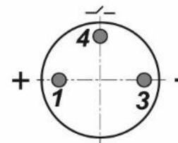
Цоколевка разъема
