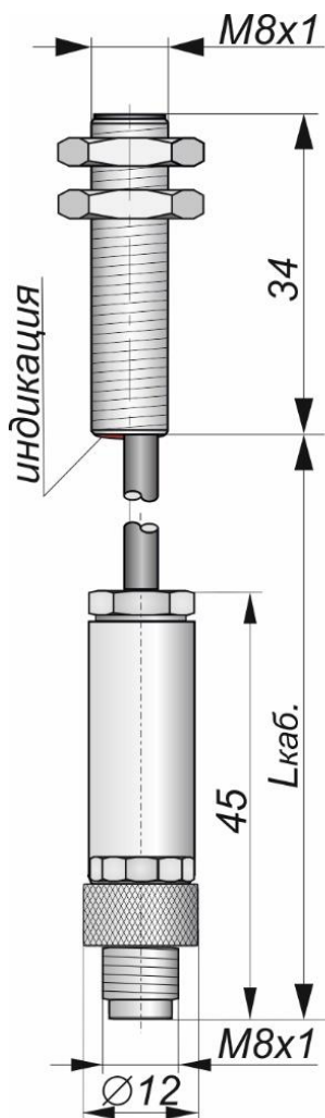
Габаритный чертеж
