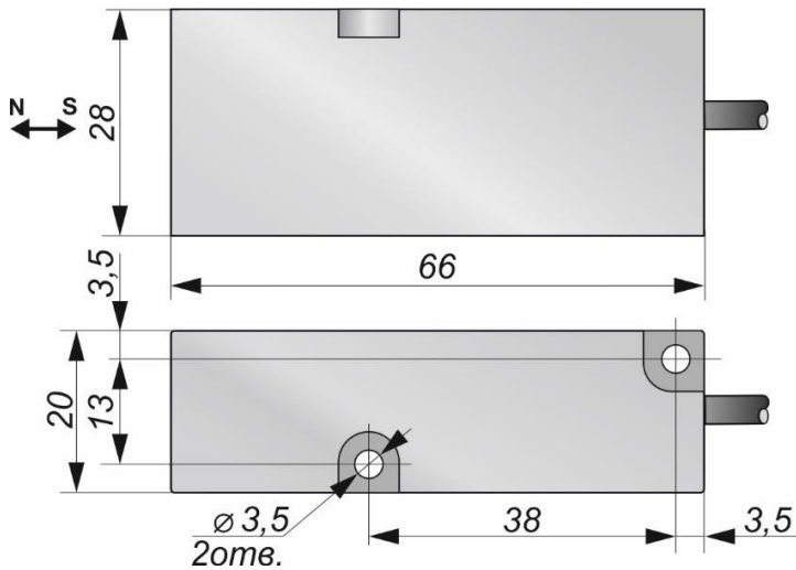
Габаритный чертеж
