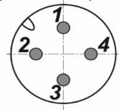
Цоколевка разъема
