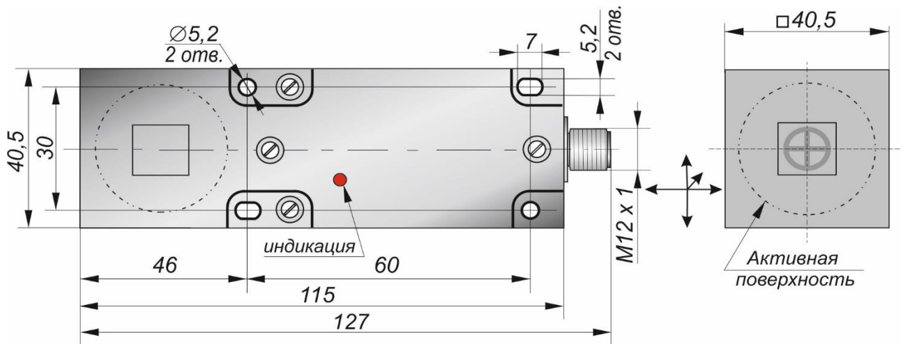
Габаритный чертеж
